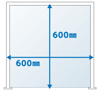
型番: FFP-HSS-66 W600×H600×D75
