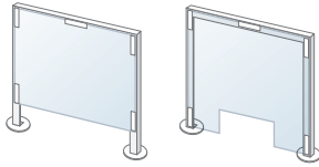
PEシートカット例(受渡し窓)
